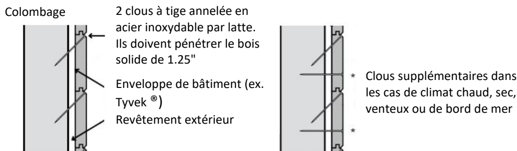
Exemple de clouage dans le cas où les fixations ne peuvent être cachées par l'embouveture
